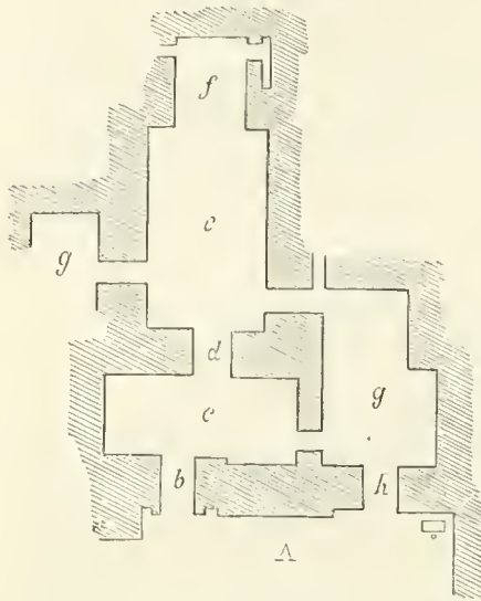
188. — Plan d'un petit temple, à Nimroud. D'après Layard.
